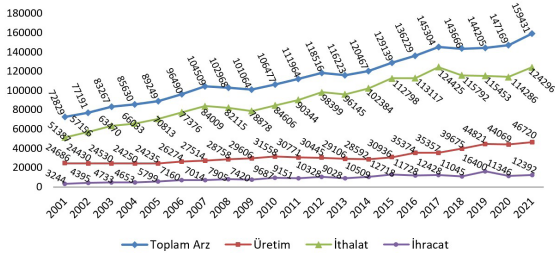
Şekil-4. 2001-2021 Türkiye Toplam Birincil Enerji Arzı, Üretimi, İthalatı, İhracatı (BinTEP)
