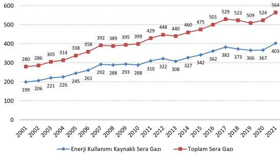
Şekil-10. 2001-2021 Toplam ve Enerji Kaynaklı Sera Gazı Miktarı (Milyon ton CO 2 eşd.)(7)
