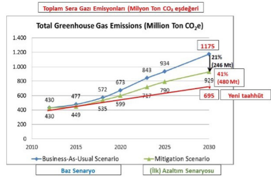
Şekil-10. Toplam Sera Gazı Emisyonları Azaltım Beyanı (Milyon Ton Co2e)(6)
